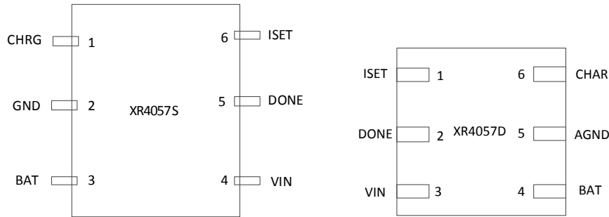
XR4057S 引脚图 (SOT23-6) 和 XR4057D 引脚图 (DFN6)
